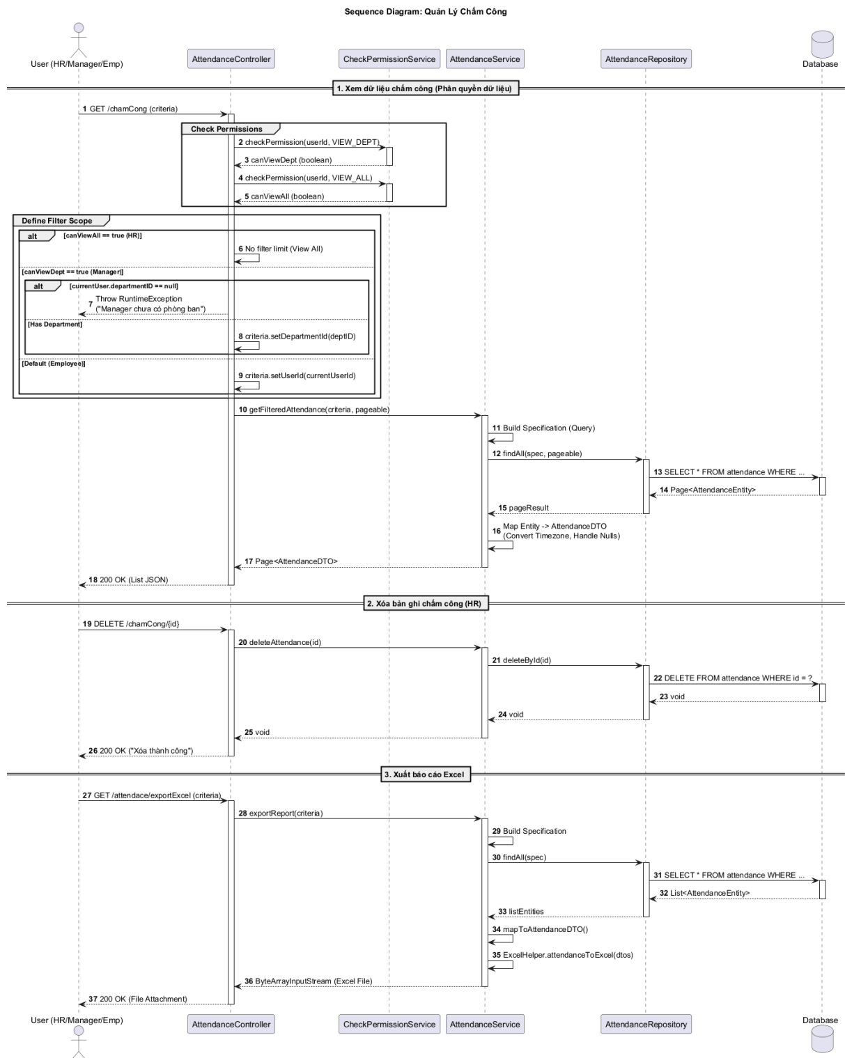
Hình 3-27: Sơ đồ tuần tự quản lý chấm công.
