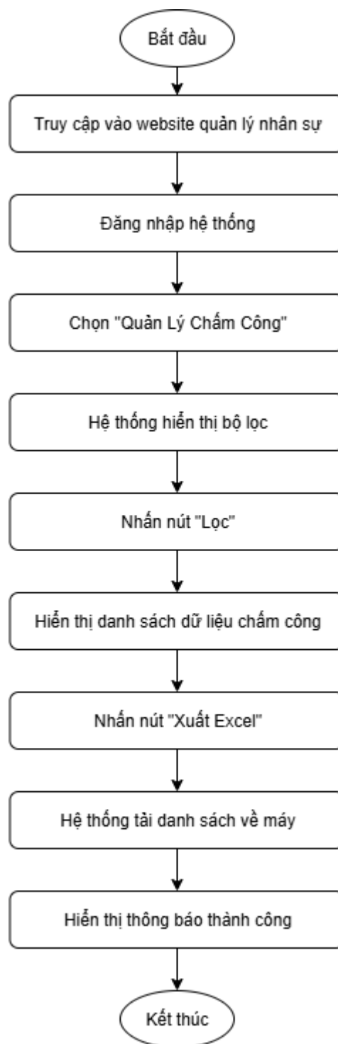
Hình 2-17: Sơ đồ quy trình Xuất file báo cáo dữ liệu chấm công.
