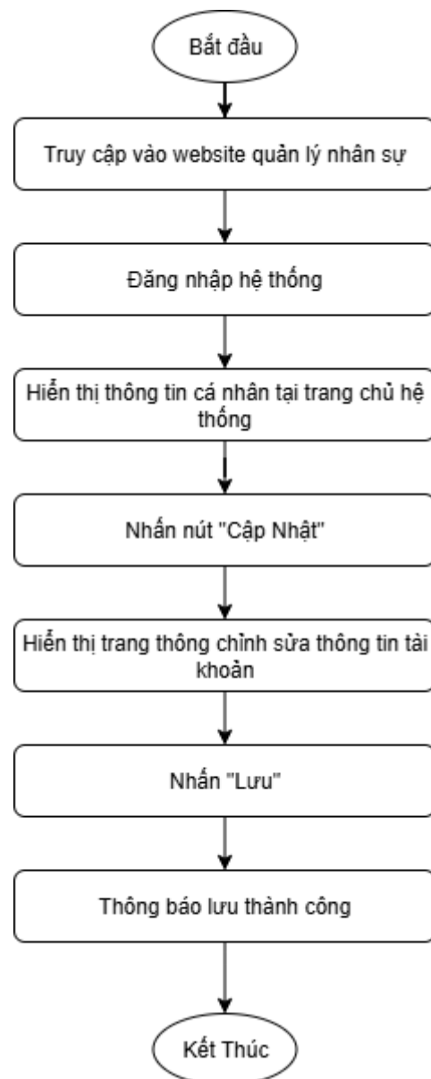
Hình 2-10: Sơ đồ quy trình Quản Lý Thông Tin Cá Nhân.
